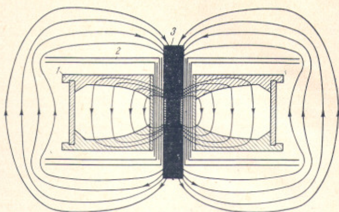
Рис. 2. Магнитная система установки Б-1. 1 — магнит, создающий постоянное магнитное поле; 2 — экраны, 3 — сердечник, создающий вихревое электрическое поле
