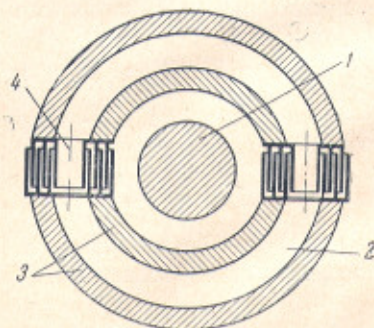
Рис. 5. Разрез камеры ускорителя СБ с лабиринтом. 1 — сердечник, создающий ускоряющее электрическое поле; 2 — экранируемый объем; 3 — стенки камеры; 4 — лабиринт
