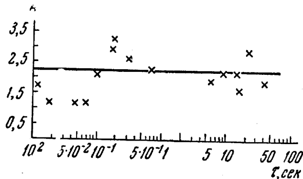
Рис. 4. Экспериментальные результаты в интервале энергий от 5 до 34 кэв и в интервале давлений от 10^{-7} до 10^{-9} мм Нг
