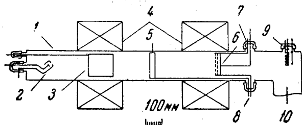
Рис. 1. Схематический разрез магнитной ловушки (в масштабе): 1 — вакуумная камера; 2 — электронная пушка; 3 — кольцо; 4 — соленоиды; 5 — электростатический зонд; 6 — коллектор; 7, 8 — сетки коллектора; 9 — манометр; 10 — к насосу
