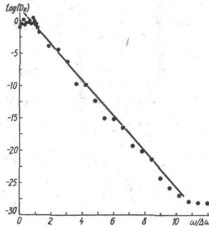
Рис. 2. Спектр корреляций D(\omega) в модуляционном стохастическом слое для модели (1): D_R = D \cdot \Delta\omega/\varepsilon^2 ; \lambda = 10 ; \omega_M = 0,01 ; \Delta\omega = 0,13 (эмпирическое значение); k = 5 \cdot 10^{-4} ; t_m = 10^6 ; s \approx 4 ; K_M \approx 40 ; V \approx 2 . Время усреднения T = 10^6 ; n = 6 . Логарифм десятичный.
