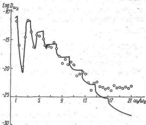
Рис. 3. Пример модуляционной диффузии в модели (8): кружки — численные данные; линия — теория (12), (13); a_1 = 0,2 ; \mu = 10^{-6} ; \varepsilon = 10^{-5} ; \Omega = 0,169 ; \lambda = 10 ; \omega_M = 0,002 ; t_m = 10^6 ; s \approx 3,5 ; K_M \approx 30 ; V \approx 2 ; T = 10^5 ; n = 4 .
